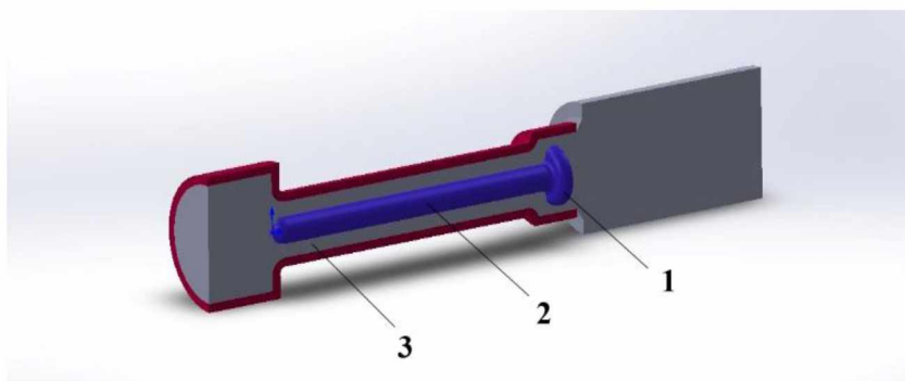
1 – дефлектор; 2 – втулка; 3 – проточный канал
